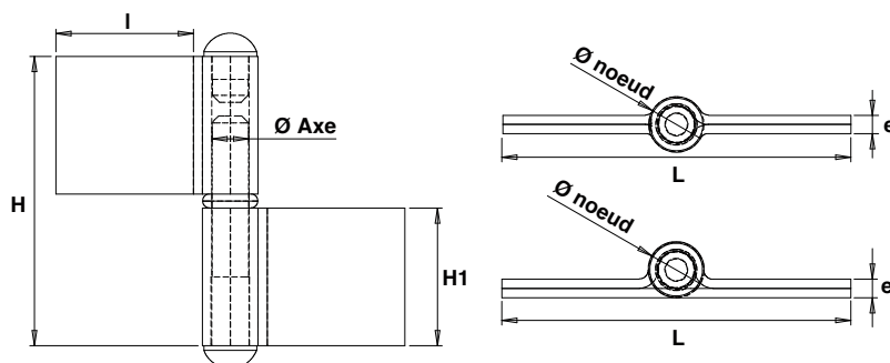
GRS.. Paumelle de grille roulée - Lames longues Lames au centre - Bague nylon
