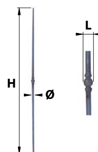
BAF27.. Barreau fantaisie 27
