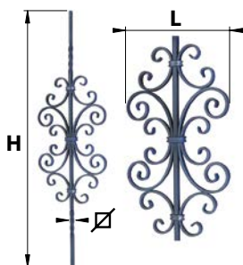
BAF22.. Barreau fantaisie 22
