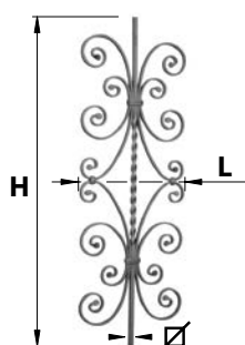
BAF92.. Barreau fantaisie 92
