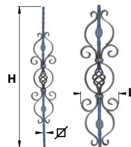
BAF37.. Barreau fantaisie 37 martelé
