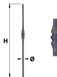
BAF148.. Barreau fantaisie 148
