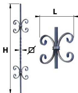
BAF10.. Barreau fantaisie double 10
