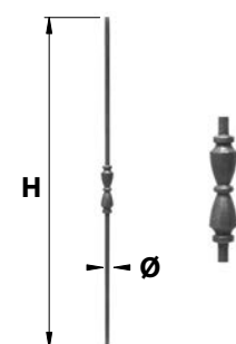
BAF125.. Barreau fantaisie 125
