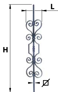
BAF90.. Barreau fantaisie 90
