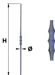
BAF118.. Barreau fantaisie 118
