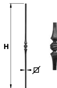
BAF144.. Barreau fantaisie 144
