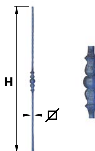
BAF66.. Barreau fantaisie 66 martelé
