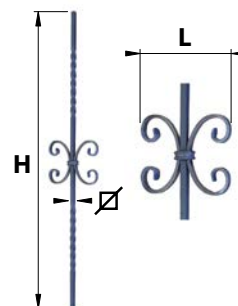
BAF09.. Barreau fantaisie 09
