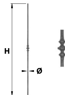
BAF128.. Barreau fantaisie 128
