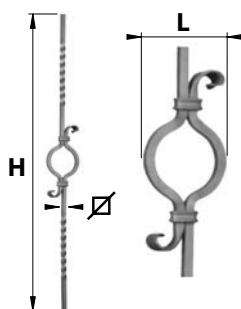
BAF34.. Barreau fantaisie torsadé 34
