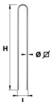
BAF45.. Barreau fantaisie 45
