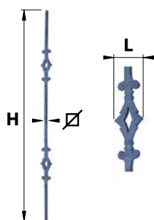
BAF30.. Barreau fantaisie double 30 martelé
