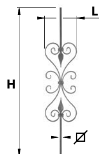
BAF83.. Barreau fantaisie 83 pointe
