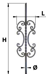
BAF20.. Barreau fantaisie 20
