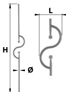
BAF86.. Barreau fantaisie 86
