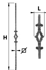
BAF29.. Barreau fantaisie 29 martelé
