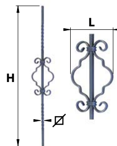
BAF07.. Barreau fantaisie 07
