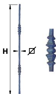
BAF47.. Barreau fantaisie double 47 martelé
