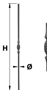
BAF71.. Barreau fantaisie 71
