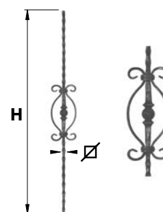
BAF123.. Barreau fantaisie 123
