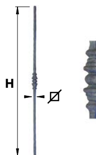
BAF46.. Barreau fantaisie 46 martelé
