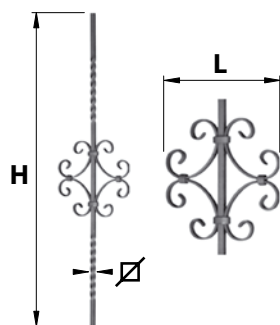
BAF16C.. Barreau fantaisie 16
