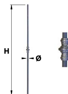
BAF111.. Barreau fantaisie double 111
