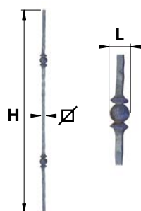
BAF24.. Barreau fantaisie 24 martelé
