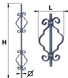
BAF08.. Barreau fantaisie double 08
