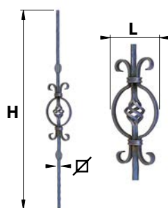
BAF36.. Barreau fantaisie 36 martelé
