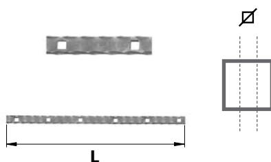
TRA55C.. Traverse 55 martelé
