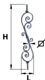
BAF77.. Barreau fantaisie 77
