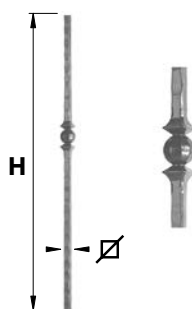
BAF58.. Barreau fantaisie 58
