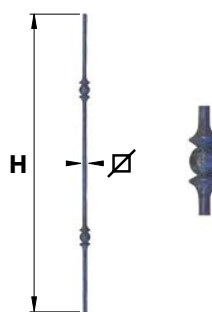
BAF135.. Barreau fantaisie double 135
