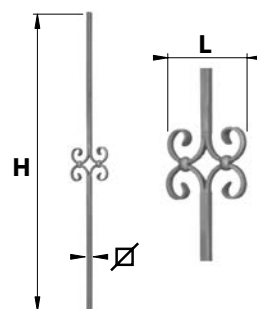
BAF02.. Barreau fantaisie 02
