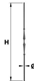
BAF140.. Barreau fantaisie 140
