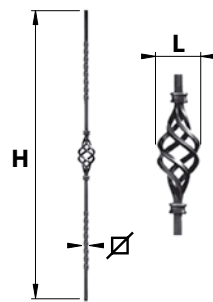
BAF05.. Barreau fantaisie 05
