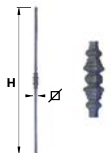
BAF46.. Barreau fantaisie 46 martelé
