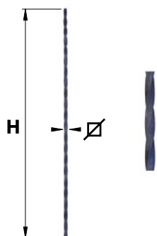
BAT58.. Barreau torsadé 58
